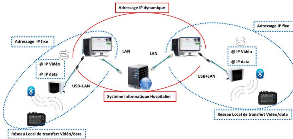
Schéma SOMNO HD/ SOMNO HD ECO avec vidéo
